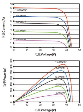
电流-电压 & 功率-电压 曲线 Current-Voltage & Power-Voltage Curve (GEP-Aa+340PH)
