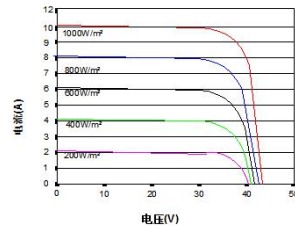
电流-电压&功率-电压 曲线 Current-Voltage & Power-Voltage Cure (GEP-De355PH)
